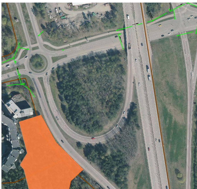
Dagvattenledningar vid korsningen Kallhällsleden/Enköpingsvägen
